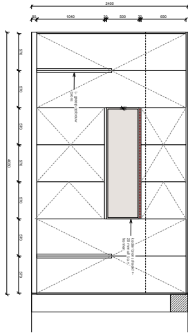
1E VERBERG | AANZICH | KASTENWAND GANG
