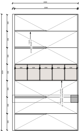
1E VERBERG | AANZICH | KASTENWAND SLAAPKAMER
