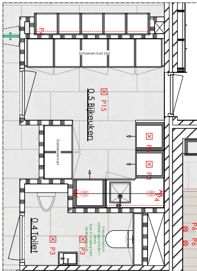
BEGANE GROND | PLATTEGROND | WERKKAMER BUKÉKEN EN TOILET
