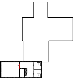
KELDER | BESTAANDE SITUATIE | SLOOP | 1:200
