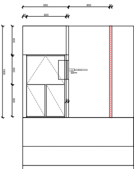
BEGANE GROND | AANZICHT | BUKÉKEN AANRECHT
