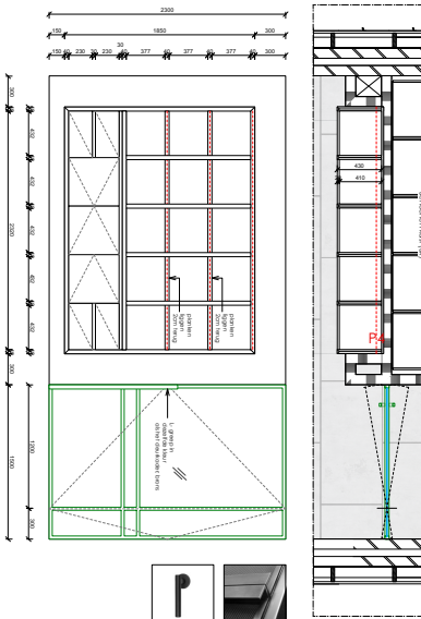
BEGANE GROND | PLATTEGROND | LANGE KASTWAND GASTENWONING
