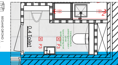
BEGANE GROND | PLATTEGROND | TOILET
