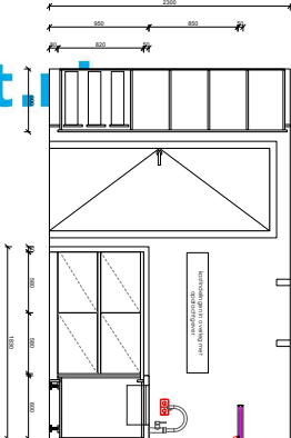
BEGANE GROND | AANZICHT | BUKÉKEN AANRECHT
