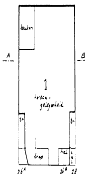
Beg grond 1:200
