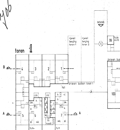
11e Verdieping 1: 200
