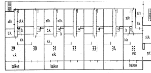
VERDIEPING 2
