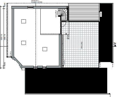
Verdieping Nieuw
