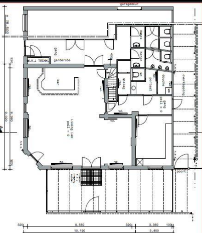
Begane grond Bestand
