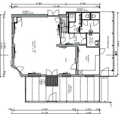
Begane grond Nieuw
