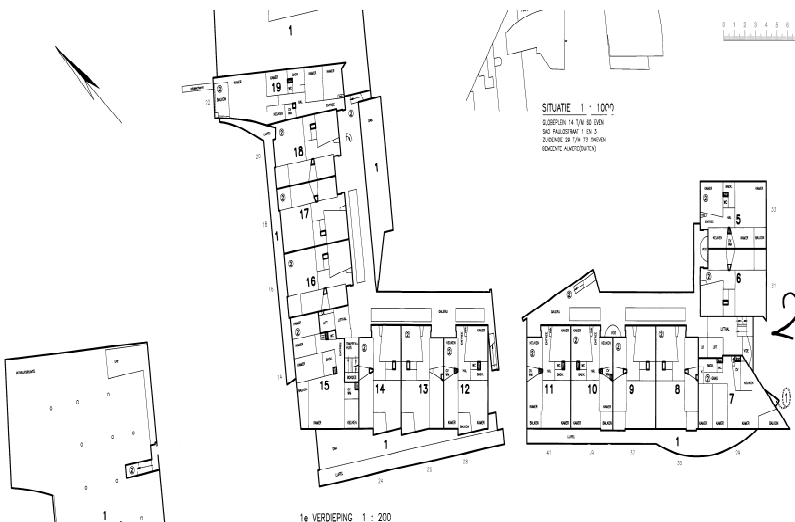
1e VERDIEPING 1 : 200
