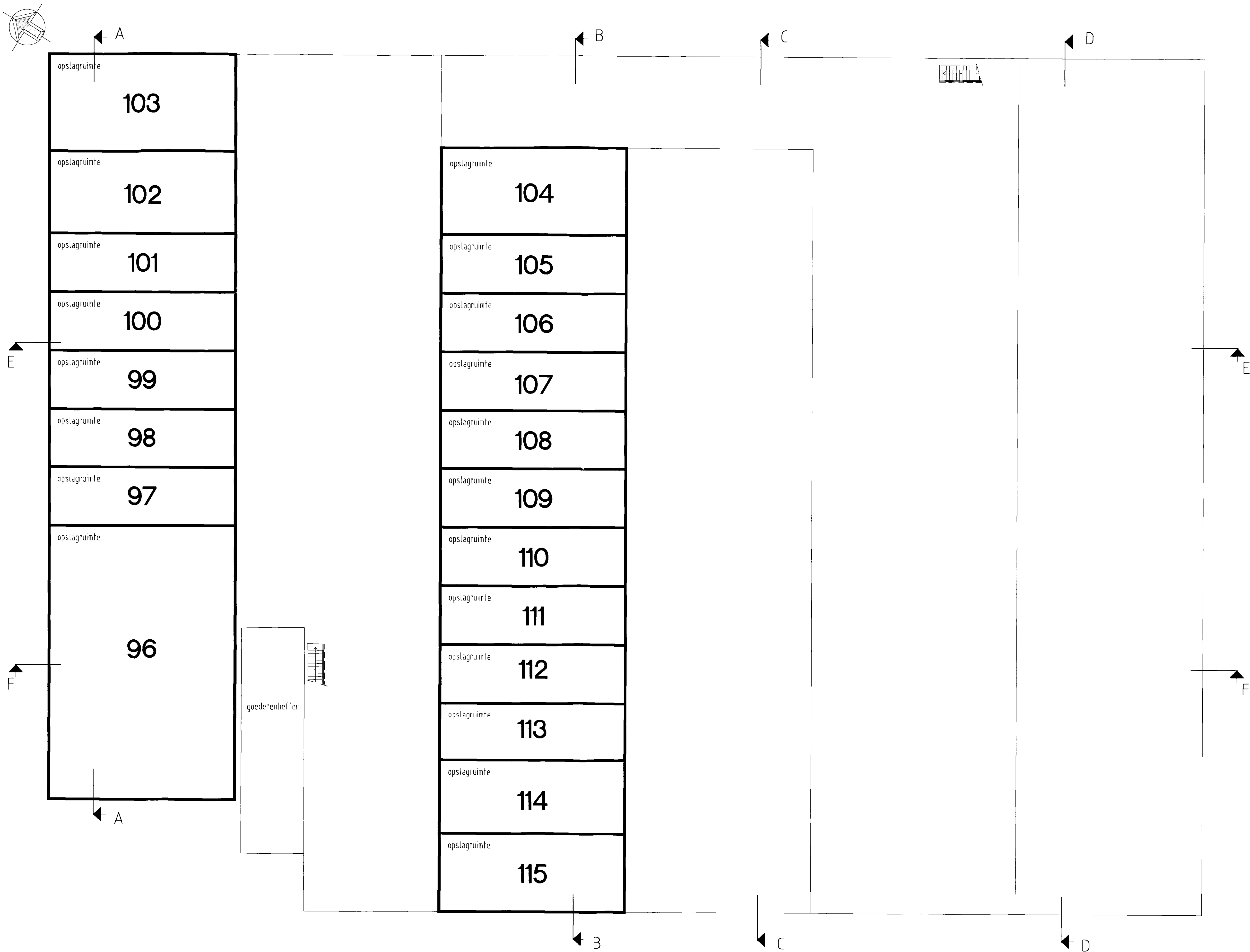
OVERZICHT 2e VERDIEPINGSVLOER OP NIVO 7820+ (schaal 1:100)
