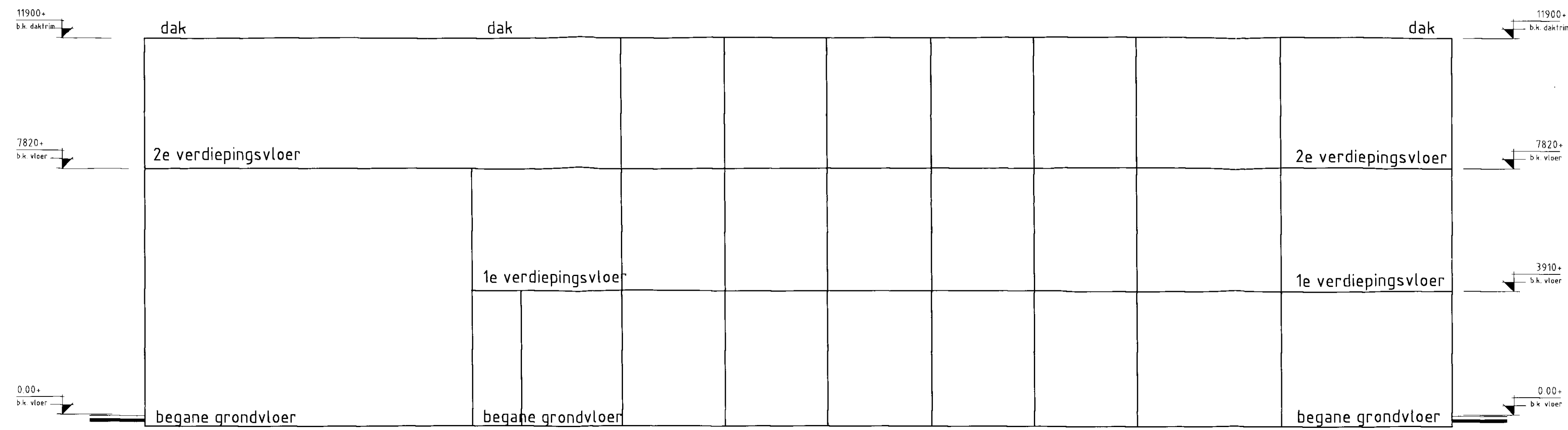
DOORSNEDE A - A (schaal 1:100)
